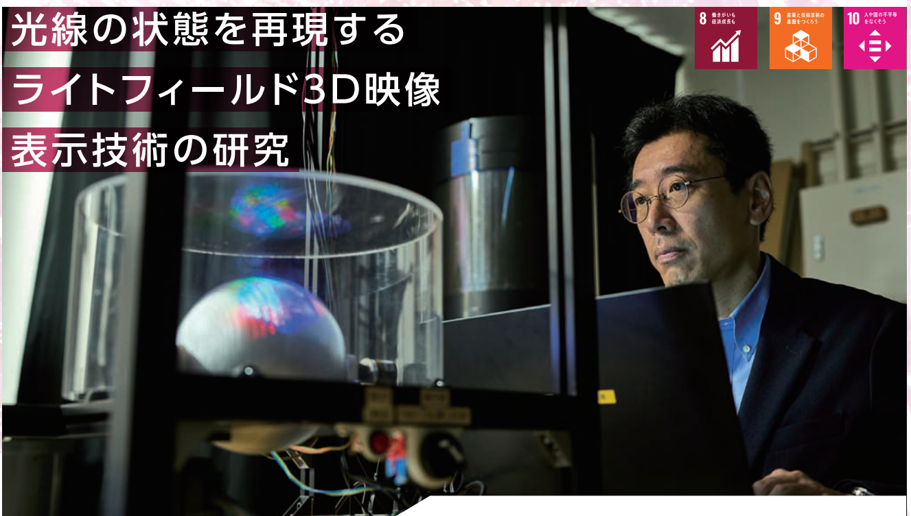
球の中に3D映像が見えるライトフィールド3Dディスプレイ。球形のため周囲の広い範囲から多人数で同時に見ることができる。
