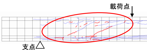
(a) 実験による橋梁の破壊状況
