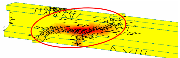
(b) 解析による橋梁の破壊状況
