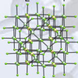
\text{Li}_2\text{MgCl}_4
