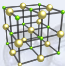
NaCl
