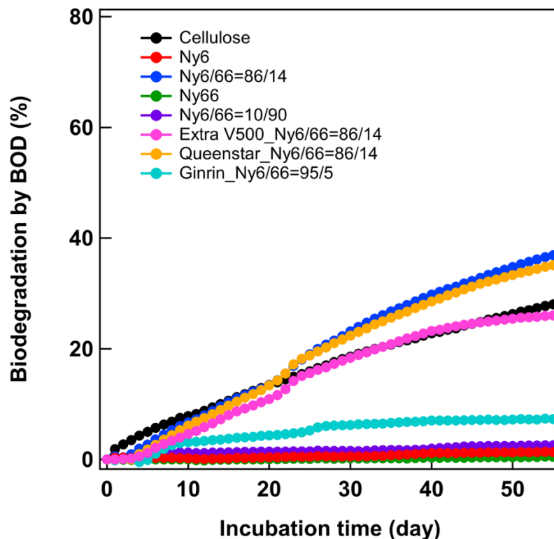
図 2 市販されているナイロン製釣り糸の生分解性（生物化学的酸素要求量；Biochemical Oxygen Demand, BOD）試験の試験結果
