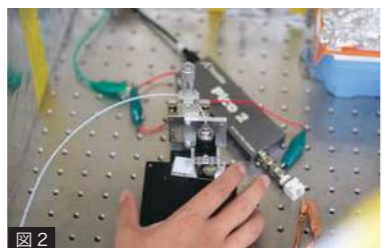
図2 人工細胞膜形成システム
