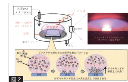
図2 気相成長法による人工ダイヤモンド成長方法
