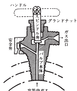
図 4－3 バルブ略図
