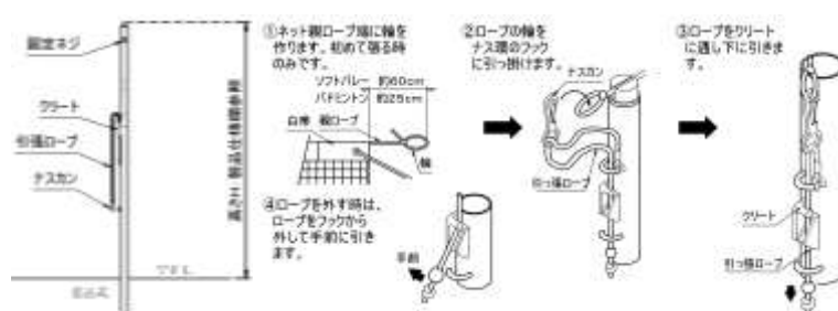
図13-5. バドミントン支柱の各部名称とネットの張り方（セノー株式会社HPより引用編集）
